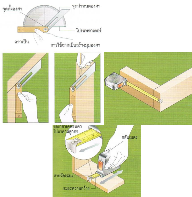
รูปที่ ๑๓ การวัดตรวจสอบความกว้างหรือความยาวด้วยตลับเมตร ที่มา: ช่างไม้ในบ้านปรับปรุง, ๒๕๕๒: หน้า ๔๓.
