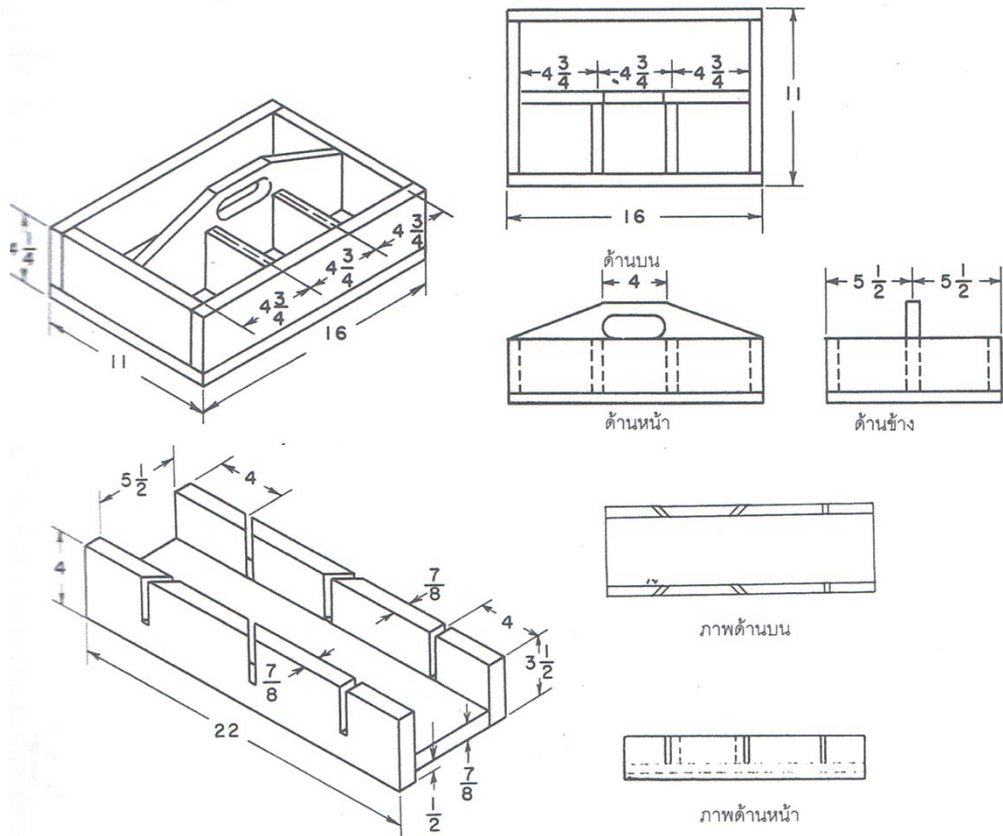
ภาพที่ ๘ แบบภาพฉายชนิดแสดง ๓ ภาพ ที่มา (เทคนิคงานไม้, ๒๕๔๐: หน้า ๓๕)
